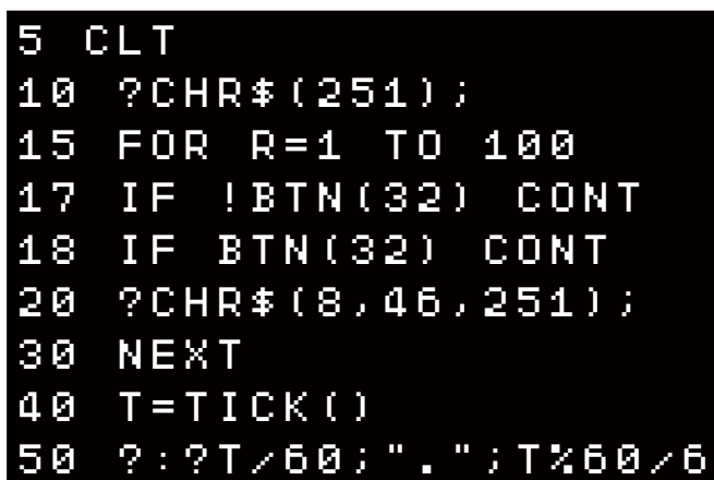
100mダッシュのプログラム
