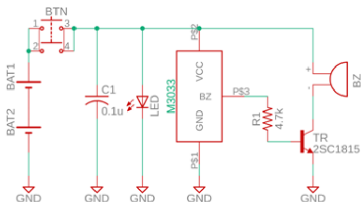
ピヨピヨブザーの回路図
